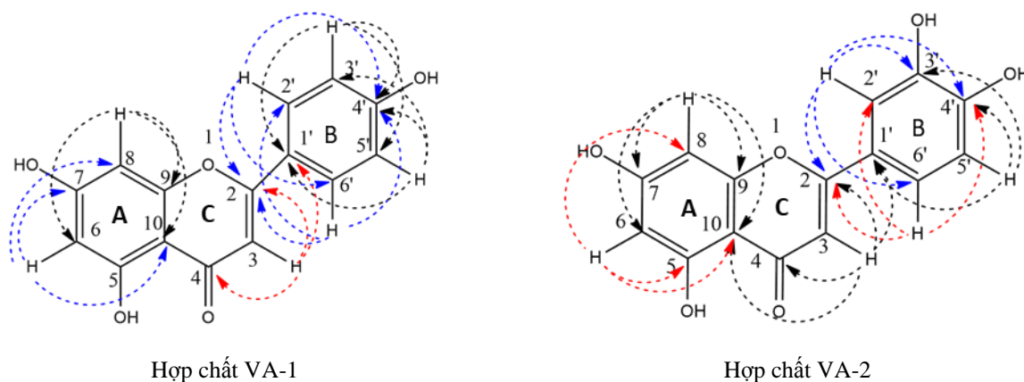
Hình 3. Cấu trúc các hợp chất VA-1 và VA-2
