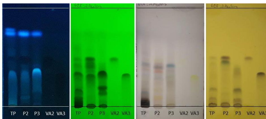
Hệ dung môi: ethyl acetat – acetone (6 : 4) Từ trái qua: UV 365 nm, UV 254 nm, TT VS, TT FeCl 3 5%/cồn
