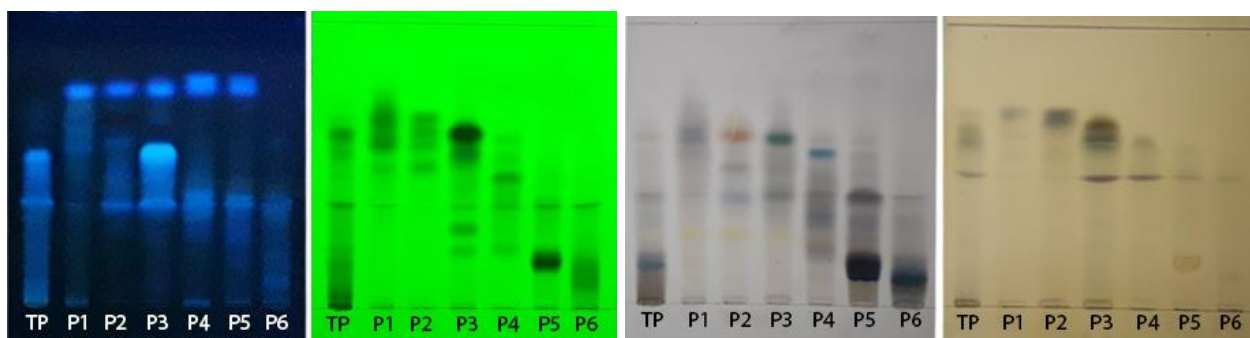
Từ trái qua: UV 365 nm, UV 254 nm, TT VS, TT FeCl 3 5%/cồn Hệ dung môi: ethyl acetat – methanol – acid formic (95: 4,5: 0,5)
